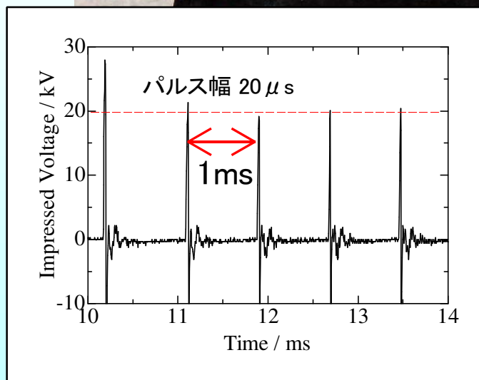
放電極距離 20mm, 放電出力4, 平均電流 80\mu\text{A}
