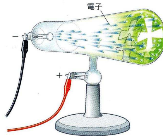
図41 十字板入り放電管と電子のモデル
